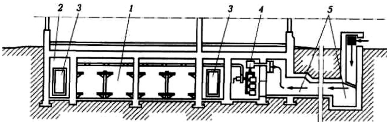
Рисунок 2 – Противорадиационное укрытие:
